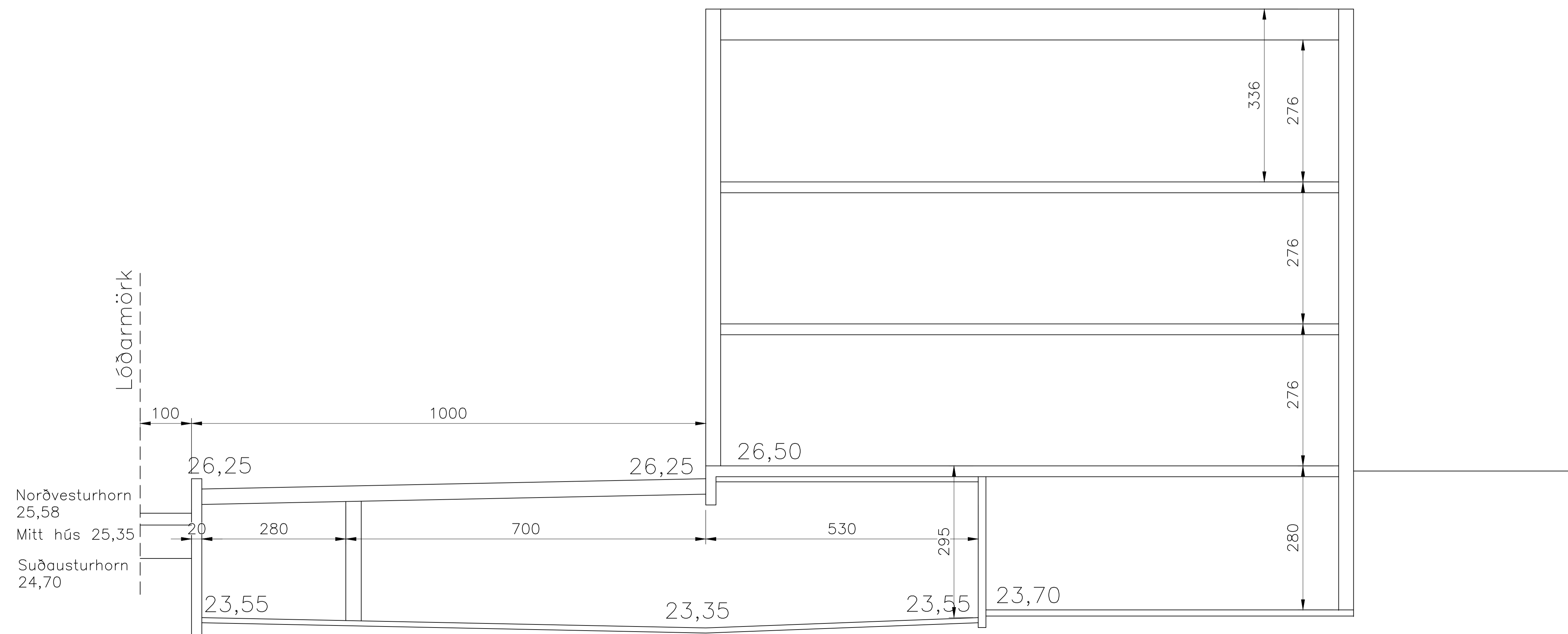
Sniðmynd í mitt hús - 1:50
